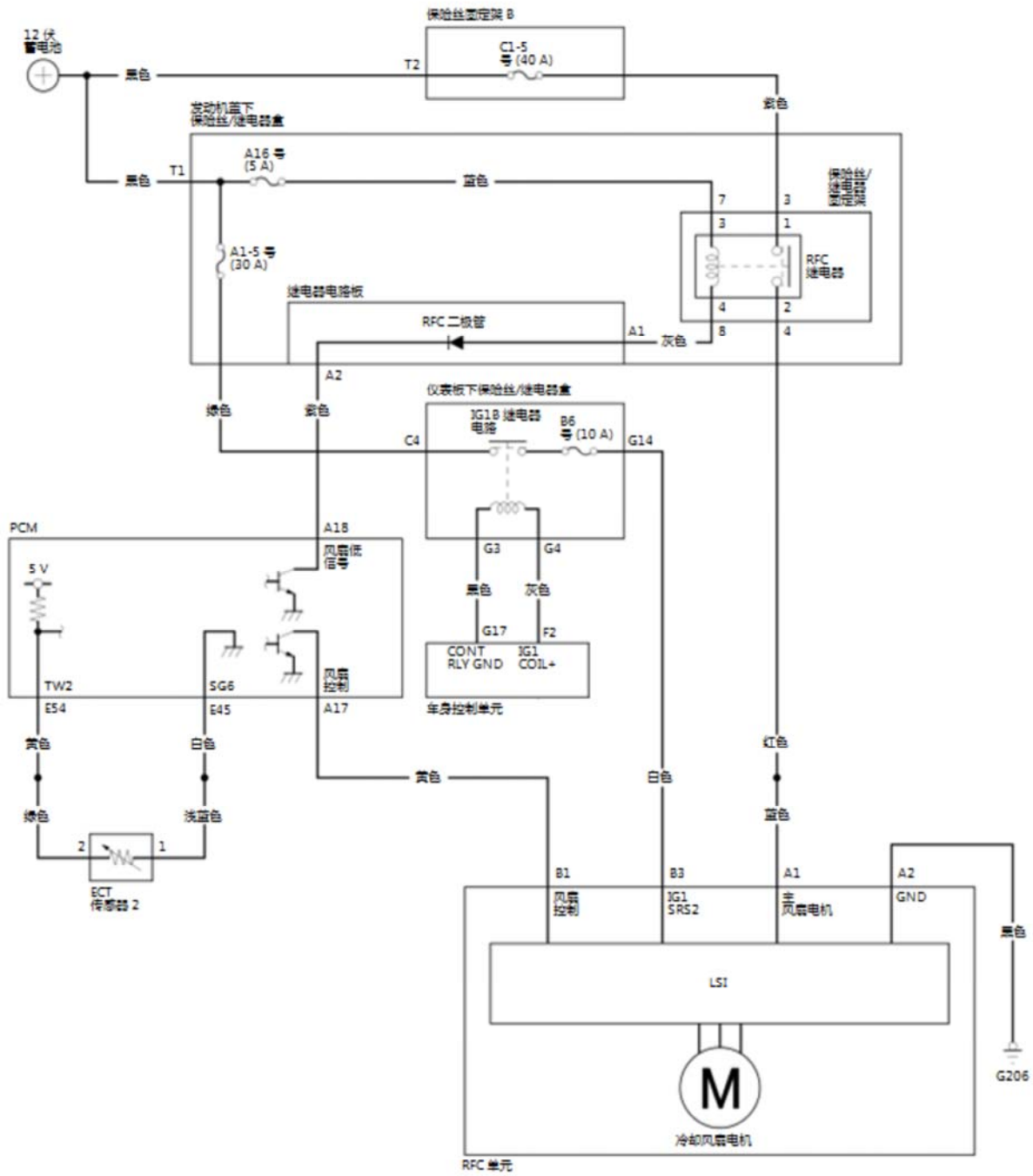
冷却风扇控制电路图
